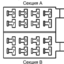
Расположение контактов разъема ISO:
